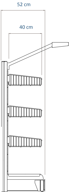
Vista Lateral
